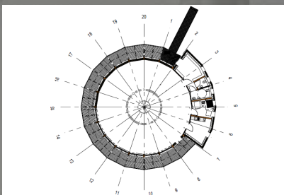
Grundriss Gebäude
