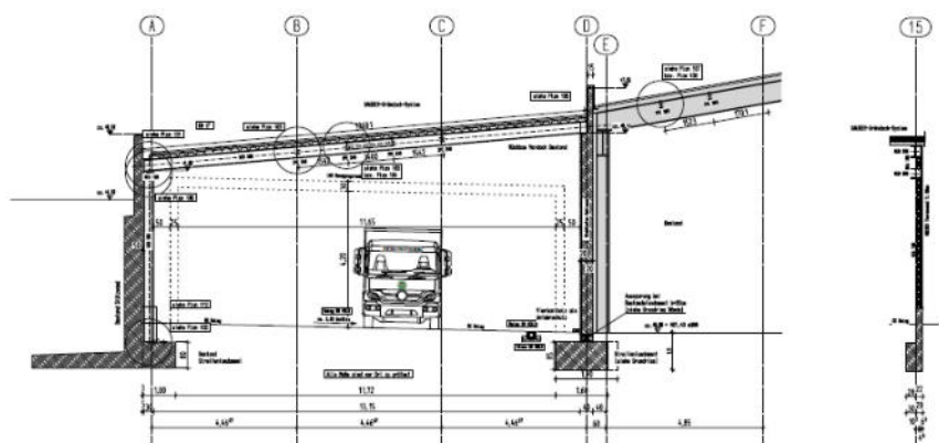
Schnitt a-a, M.: 1:50
